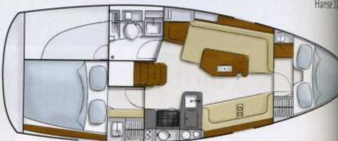
Hanse 630
